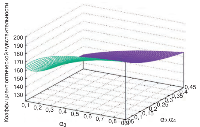
Рис. 6. Трехмерный график зависимости C_G при изменяющихся молярных долях \alpha_2, \alpha_3, \alpha_4 , при \alpha_2=\alpha_4
