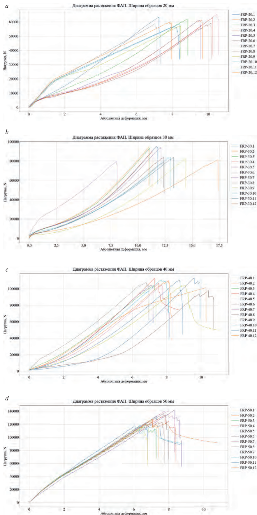
Рис. 3. Диаграмма нагружения образцов серии: а – FRP-20; б – FRP-30; в – FRP-40; д – FRP-50 Fig. 3. Loading diagram for specimens of the series: а – FRP-20; б – FRP-30; в – FRP-40; д – FRP-50
