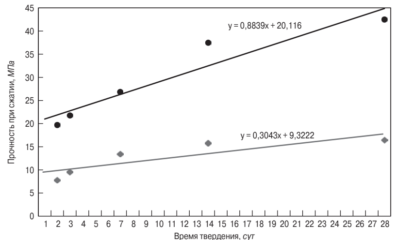
Рис. 3. Кинетика набора прочности композиционного вяжущего: ● – 15% технического углерода; ◆ – 30% технического углерода Fig. 3. Kinetics of strength development of the composite binder: ● – 15% carbon black; ◆ – 30% carbon black
