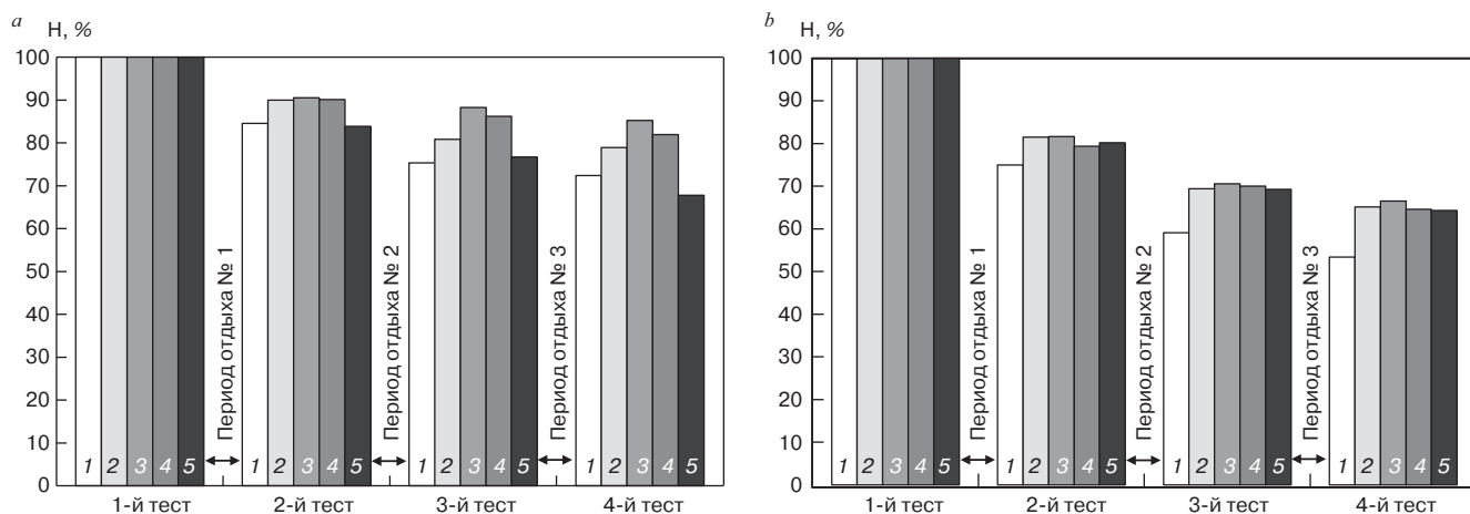
Рис. 8. Изменение прочности ЦМА после повторных испытаний при сжатии с различным содержанием капсул на основе подсолнечного масла (a) и AR-полимера (b): 1 – без капсул; 2 – 1,5%; 3 – 3%; 4 – 4,5%; 5 – 9%
