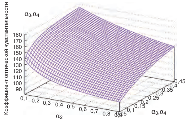
Рис. 5. Трехмерный график зависимости C_G при изменяющихся молярных долях \alpha_2, \alpha_3, \alpha_4 , при \alpha_3=\alpha_4
