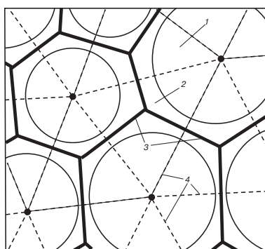
Рис. 2. Геометрия структуры на примере ячеистого материала: 1 — поры (ячейки) в материале; 2 — межпоровые перегородки; 3 — расположение осей каркаса; 4 — расположение осей конвективных потоков Fig. 2. Geometry of the structure on the example of a cellular material): 1 — pores (cells) in the material; 2 — interpore partitions; 3 — location of the axes of the frame; 4 — the location of the axes of convective flows
