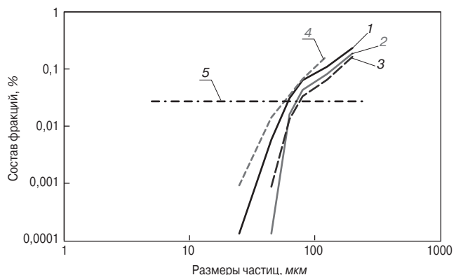
Рис. 5. Распределение Розина-Раммлера частиц цемента с разной энергией активации: 1 – контрольный цемент; 2 – цемент с энергией активации 17 кДж/кг; 3 – цемент с энергией активации 34 кДж/кг; 4 – цемент с энергией активации 51 кДж/кг; 5 – R=36,8%
