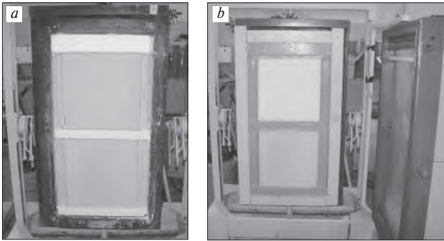
Рис. 1. Испытания фрагментов бетонных плит с нанесенными составами облицовочно-декоративных систем по бетонному основанию (а) и по керамической плитке (б) в холодильно-дождевальной установке ХДУ-02 «Термоизоляция»
