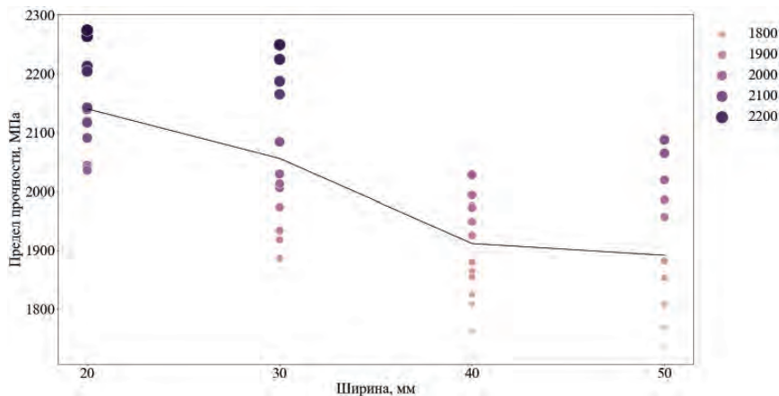
Рис. 1. Распределение значений сопротивления ФАП ламината при изменении ширины образца Fig. 1. Distribution of resistance values of FRP laminate when changing the width of the sample
