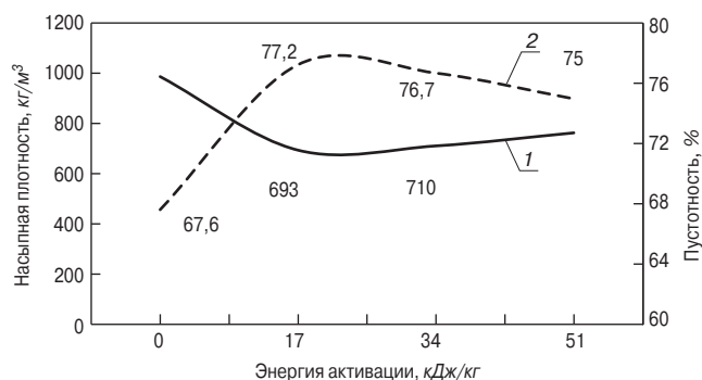
Рис. 2. Изменение агломерации частиц цемента с различной энергией активации: 1 – насыпная плотность; 2 – пустотность
