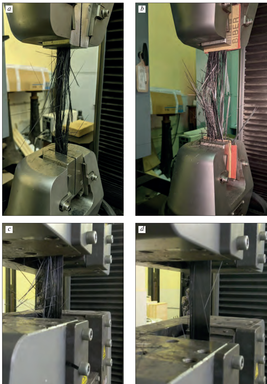
Рис. 3. Разрушение образцов серии: а – FRP-20; б – FRP-30; в – FRP-40; д – FRP-50 Fig. 3. Destruction of samples of the series: а – FRP-20; б – FRP-30; в – FRP-40; д – FRP-50
