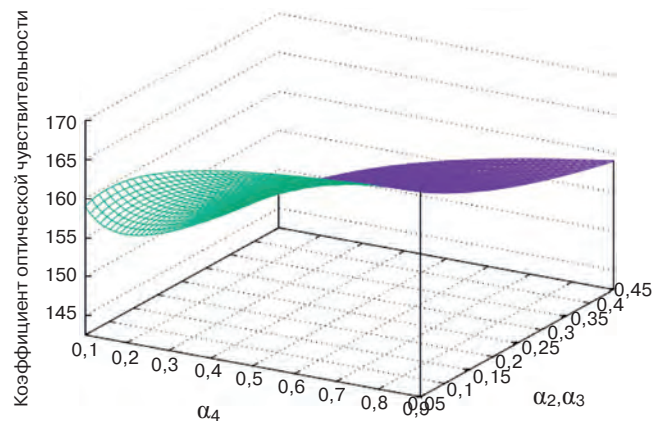
Рис. 7. Трехмерный график зависимости C_G при изменяющихся молярных долях \alpha_2, \alpha_3, \alpha_4 , при \alpha_2=\alpha_3
